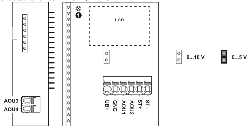
Aansluitschema voor 22DC-..1, 22DTC-..1
